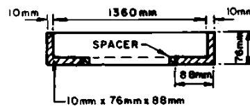
SECTION A-A "FRAME"
